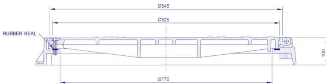
SECTION A-A
