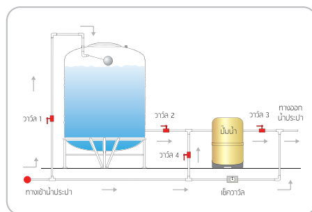
การติดตั้งประปา 3 ระบบ
