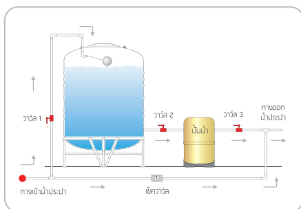
การติดตั้งประปา 2 ระบบ
