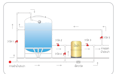
การติดตั้งประปา 4 ระบบ
